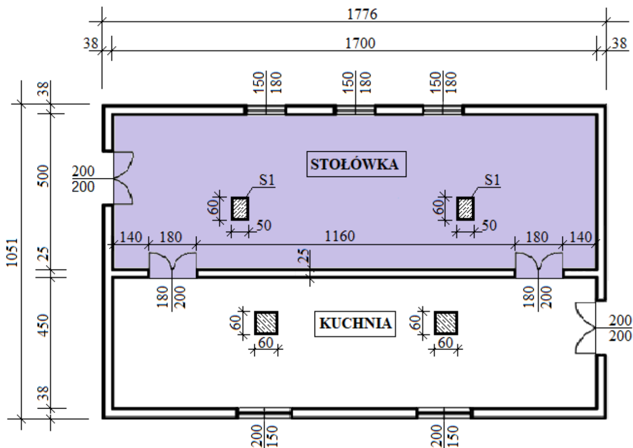
Rzut kuchni i stołówki
