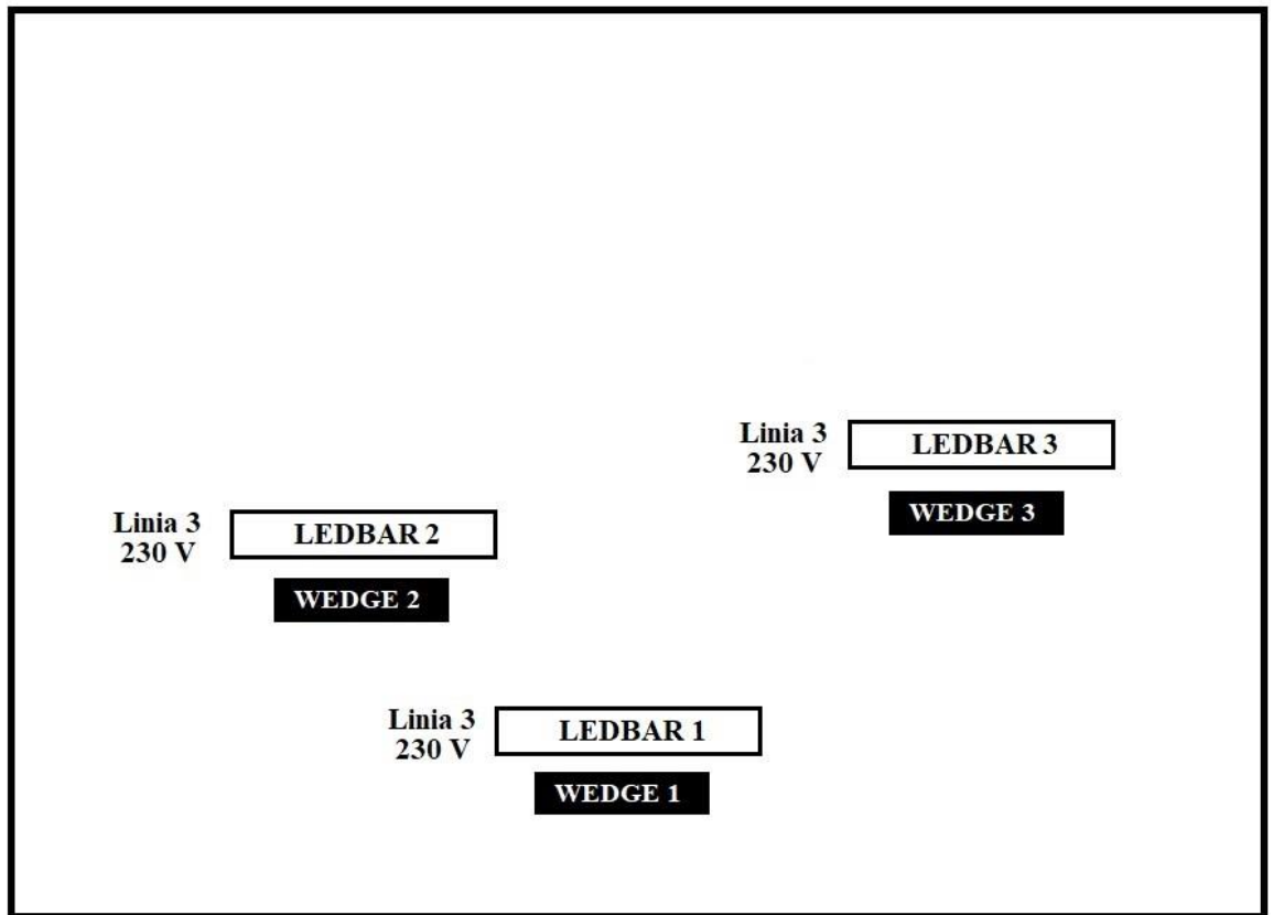
Rysunek 2. Plan sceny dla światła
