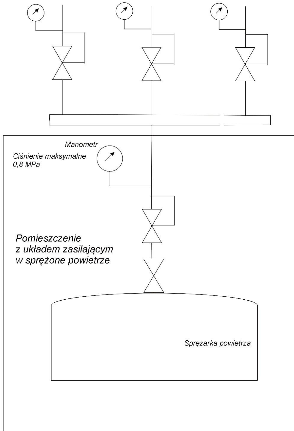
Rysunek 2. Schemat instalacji sprężonego powietrza
