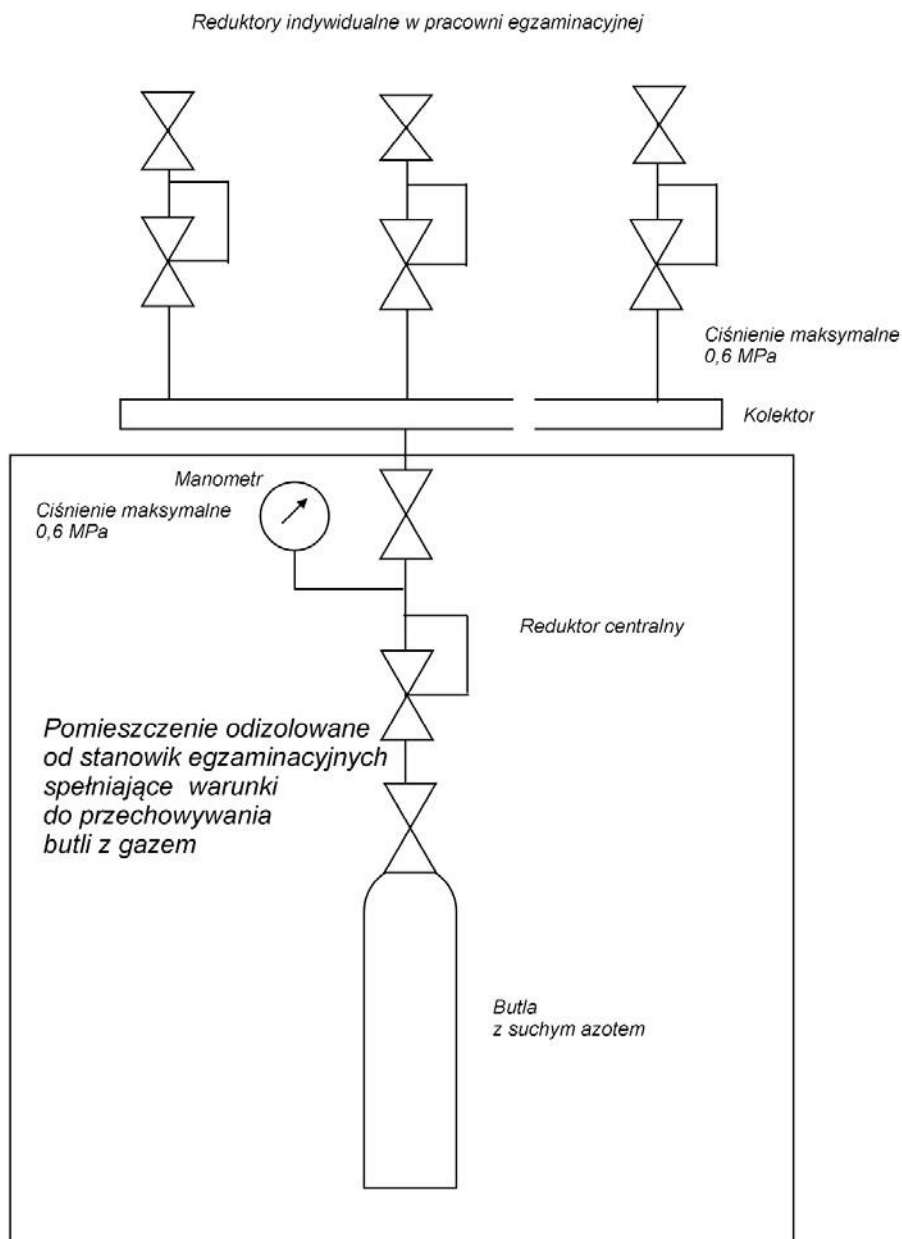
Rysunek 2. Schemat instalacji gazowej
