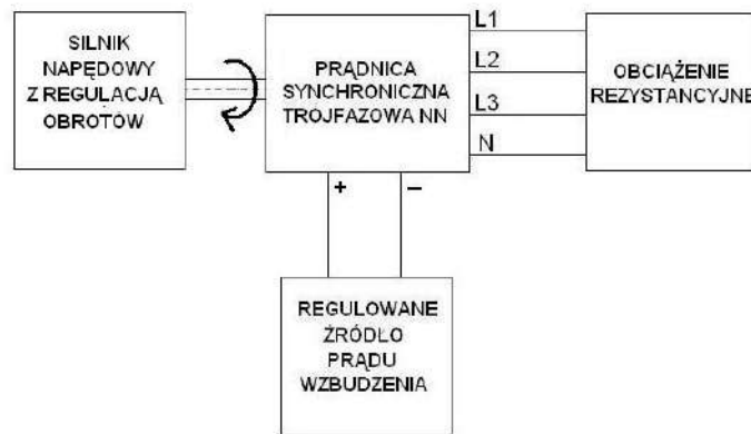
Rysunek 1. Schemat blokowy układu pomiarowego prądnicy synchronicznej
