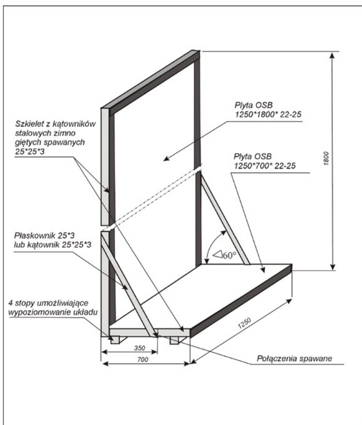
Rysunek 1. Konstrukcja stanowiska egzaminacyjnego
